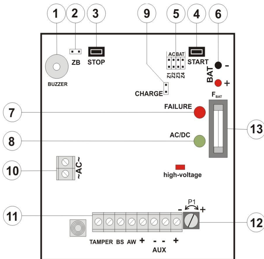
Rys. 2. Widok płyty pcb zasilacza.
