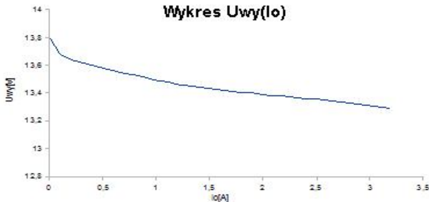
Rys.4. Wykres U_{wy} = f(I_o) .
