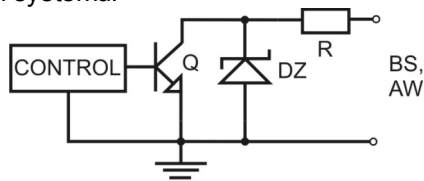
Rys. 6. Schemat elektryczny wyjść OC.
