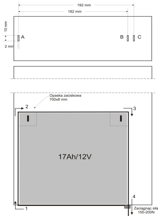
Rys.5. Procedura mocowania akumulatora.
