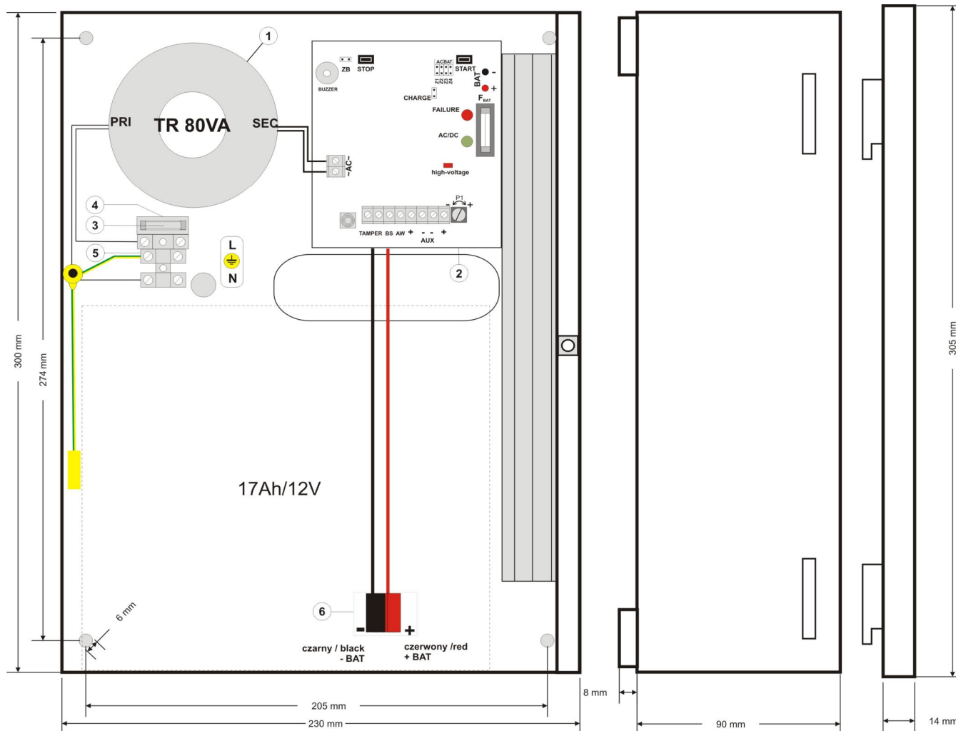
Rys.3. Widok zasilacza.
