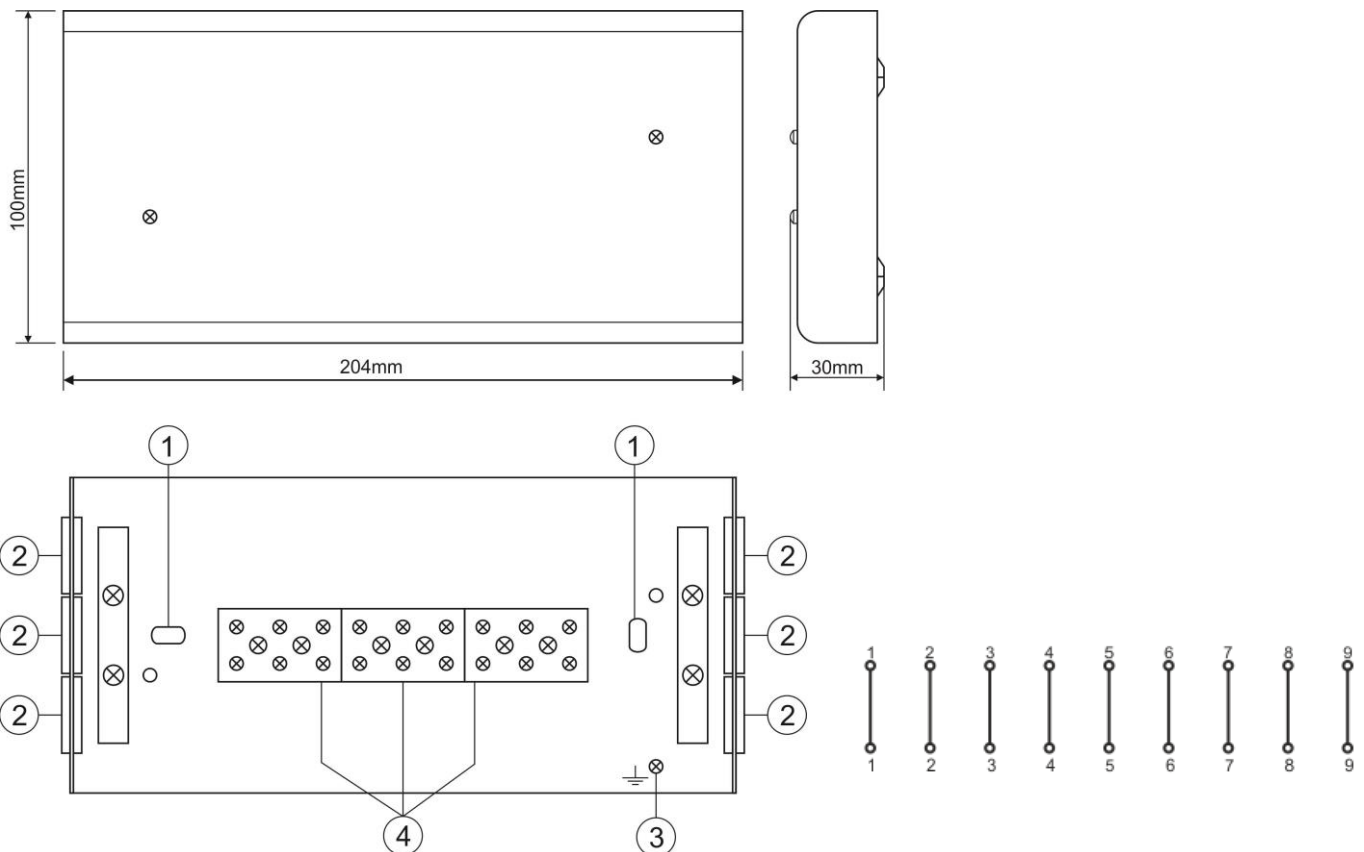
Rys.1. Widok puszki instalacyjnej.
