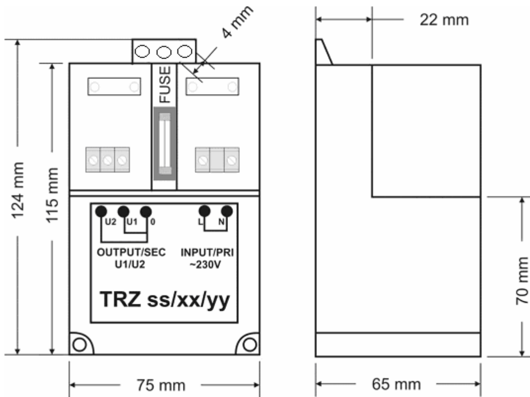
Fig.1 TRZ 20/U1/U2 ÷ TRZ 60/U1/U2
