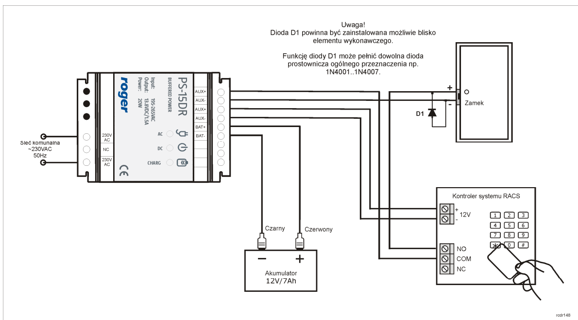
Rys.4 Przykład wykorzystania zasilacza w systemie kontroli dostępu
