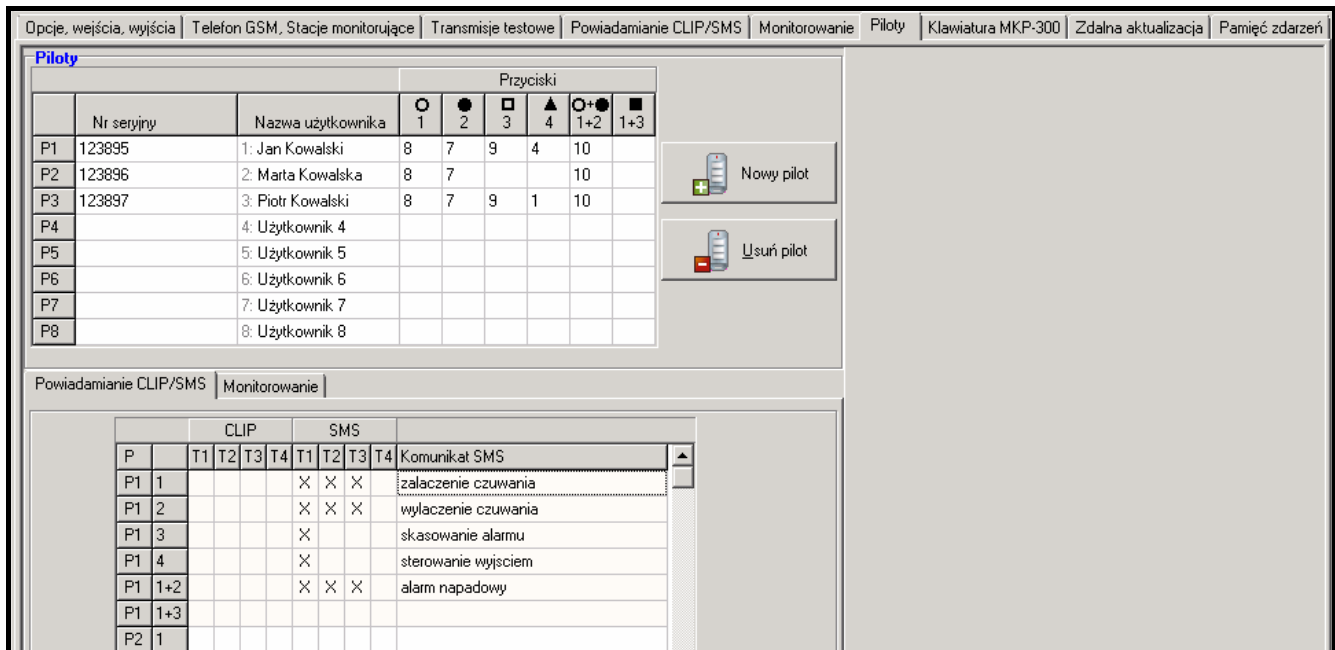
Rys. 15. Zakładka „Piloty”.
